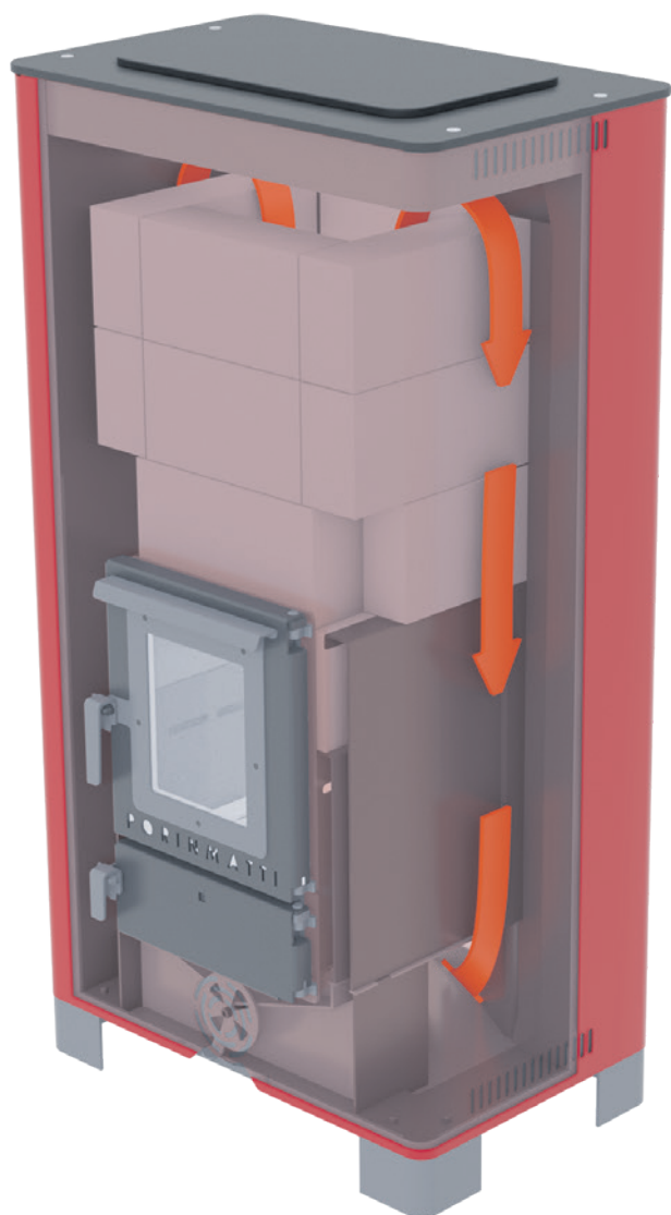
Värmekanaler
